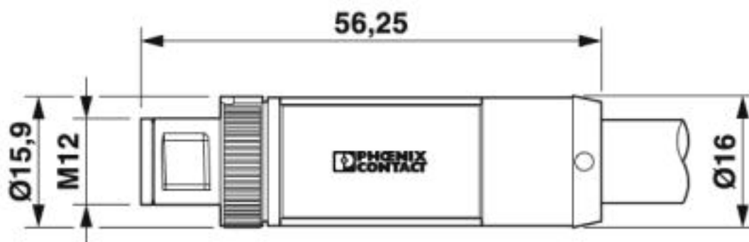
Maßzeichnung
