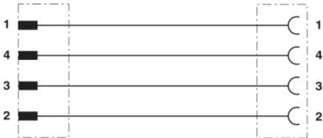
Schaltplan
