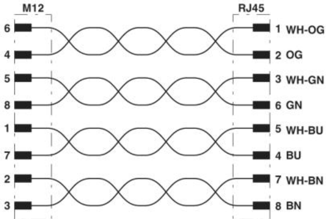
Schaltplan
