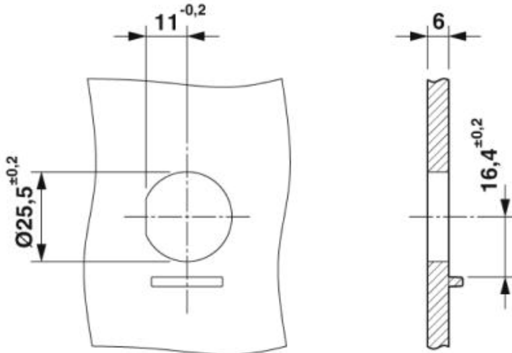
Maßzeichnung
