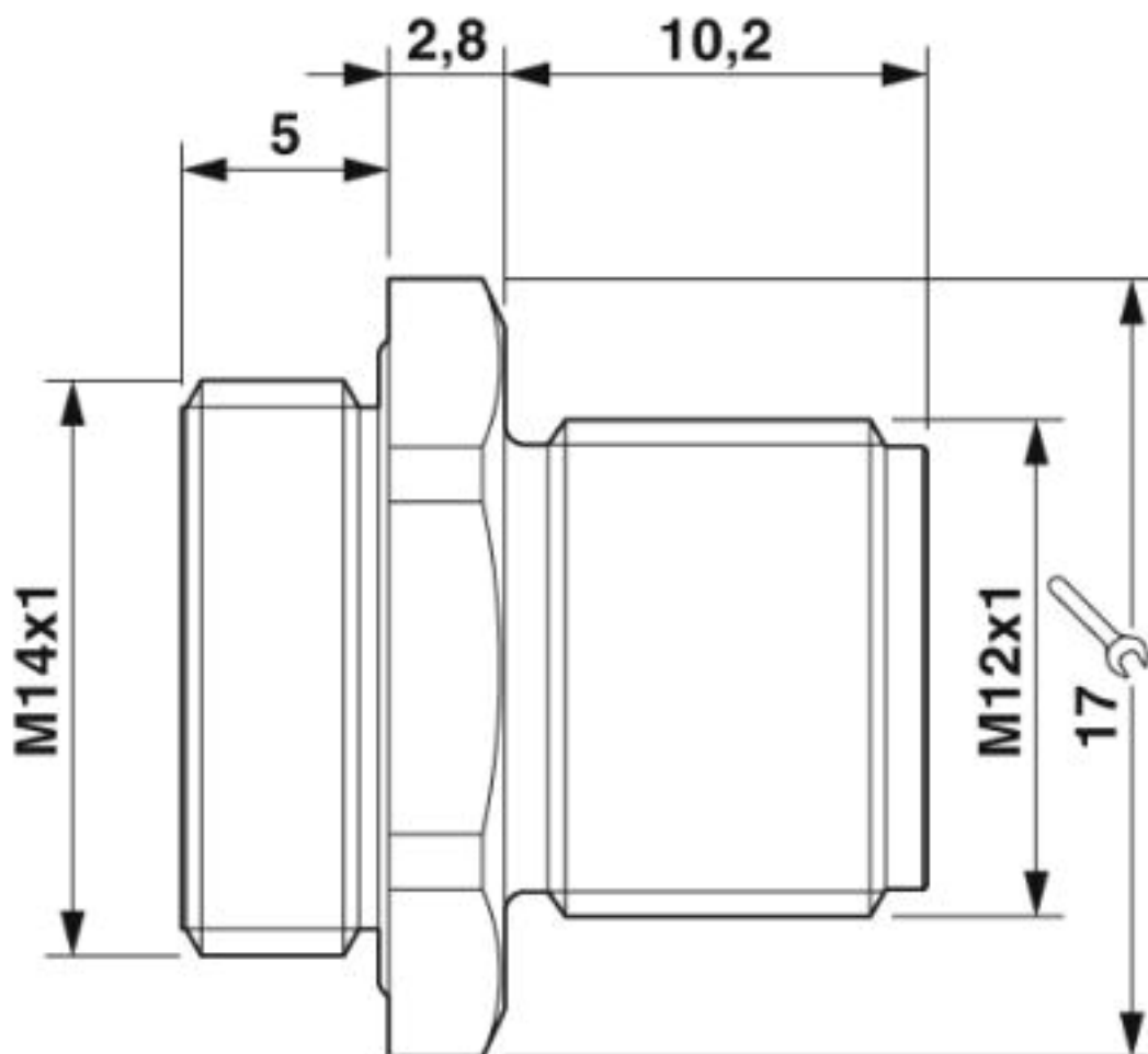
Maßzeichnung
