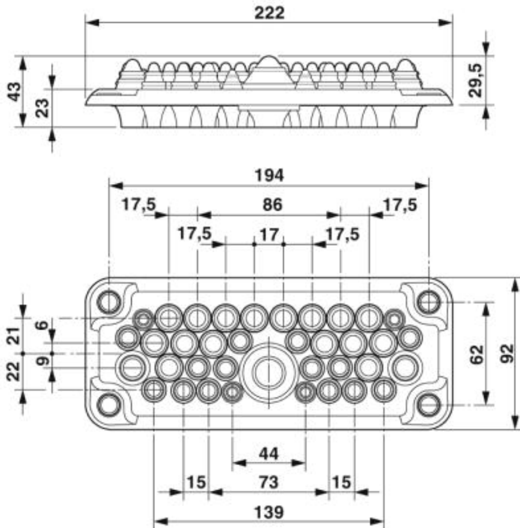
Maßzeichnung
