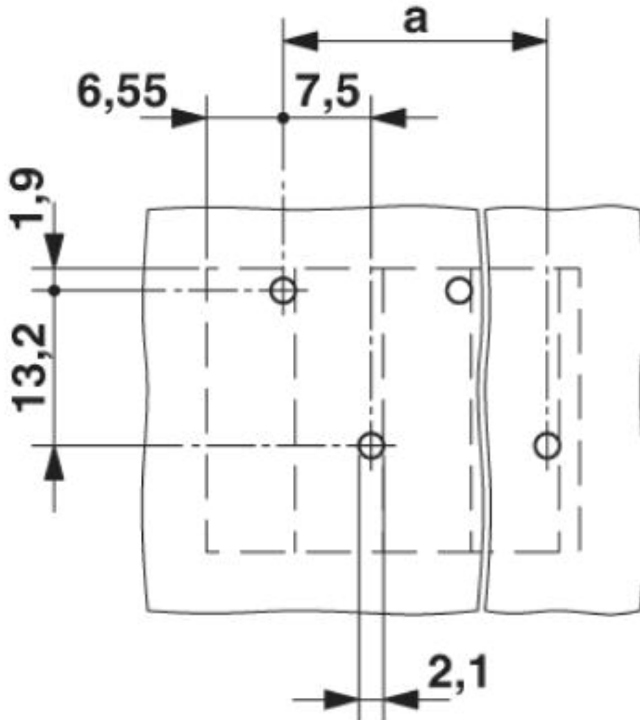
Bohrplan
