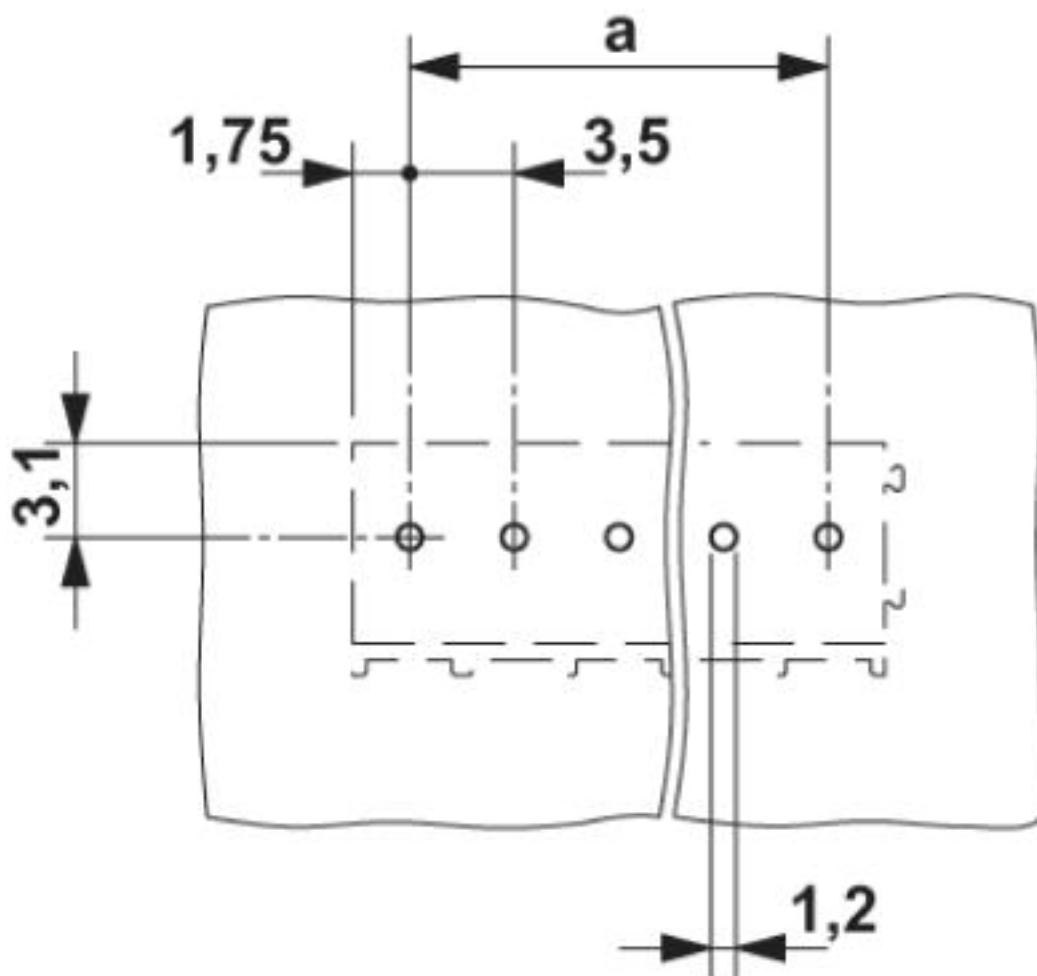
Bohrplan
