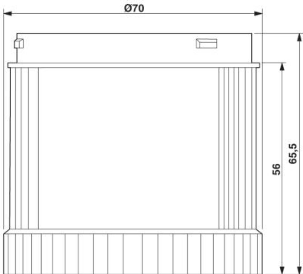
Maßzeichnung
