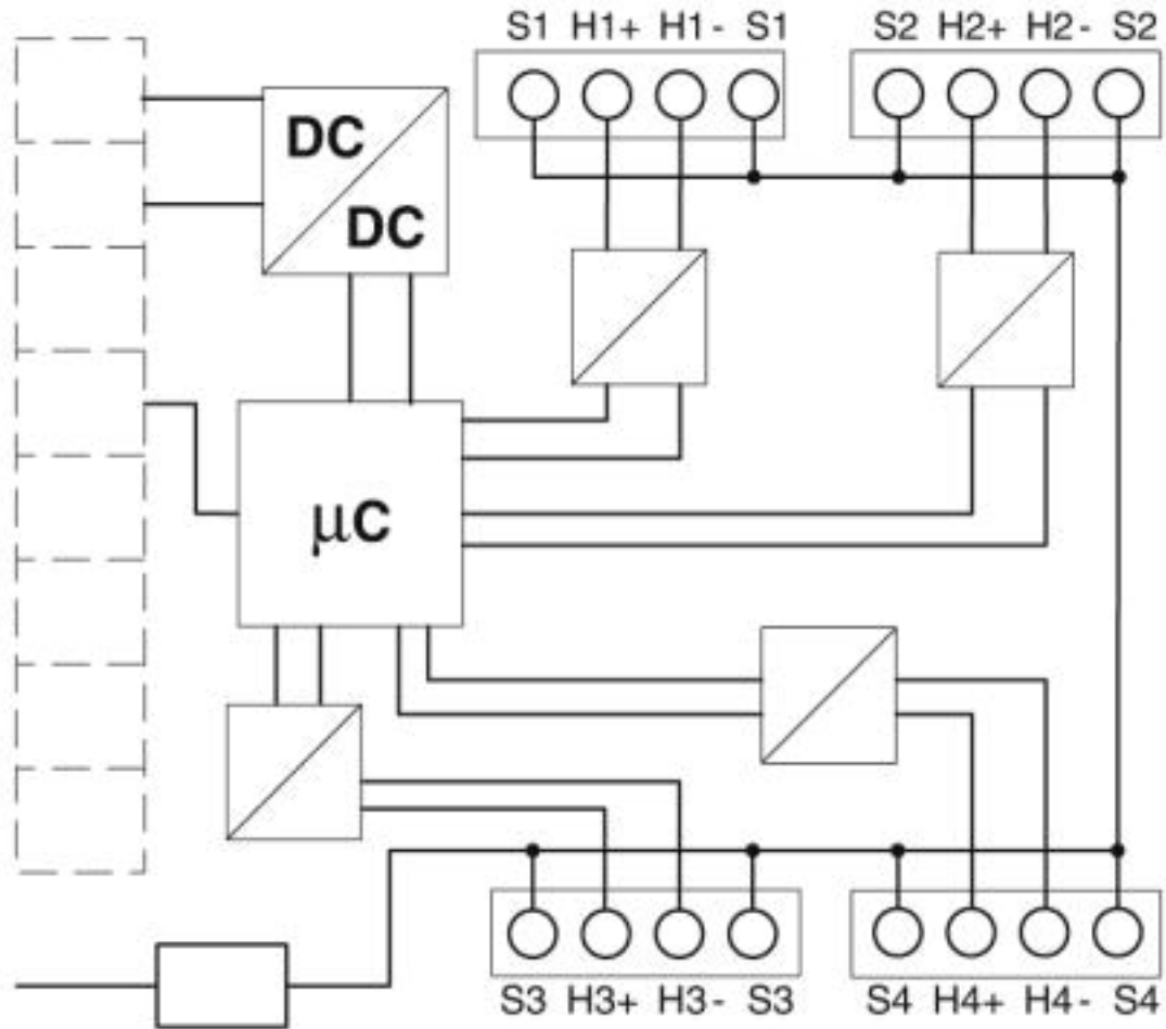
Blockschaltbild
