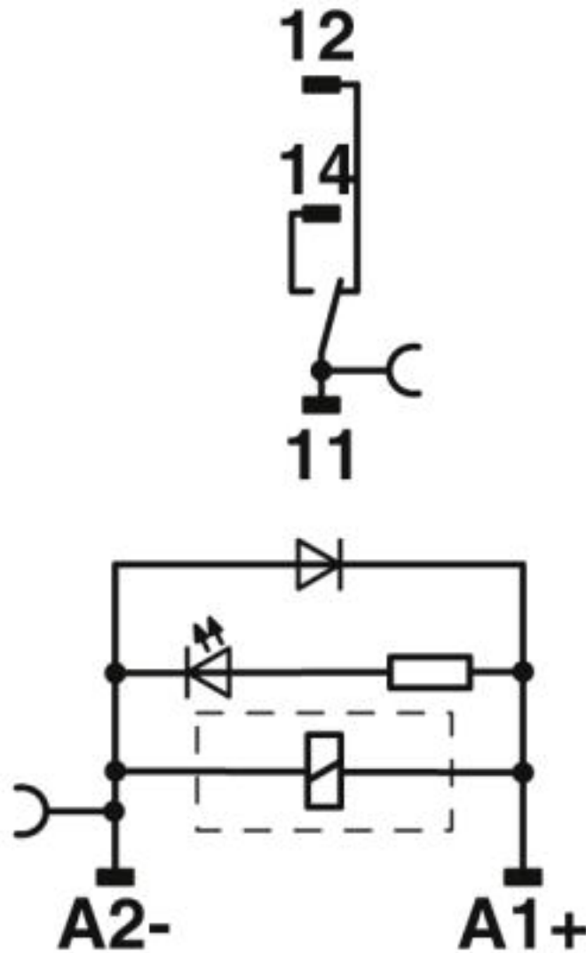
Schaltplan
