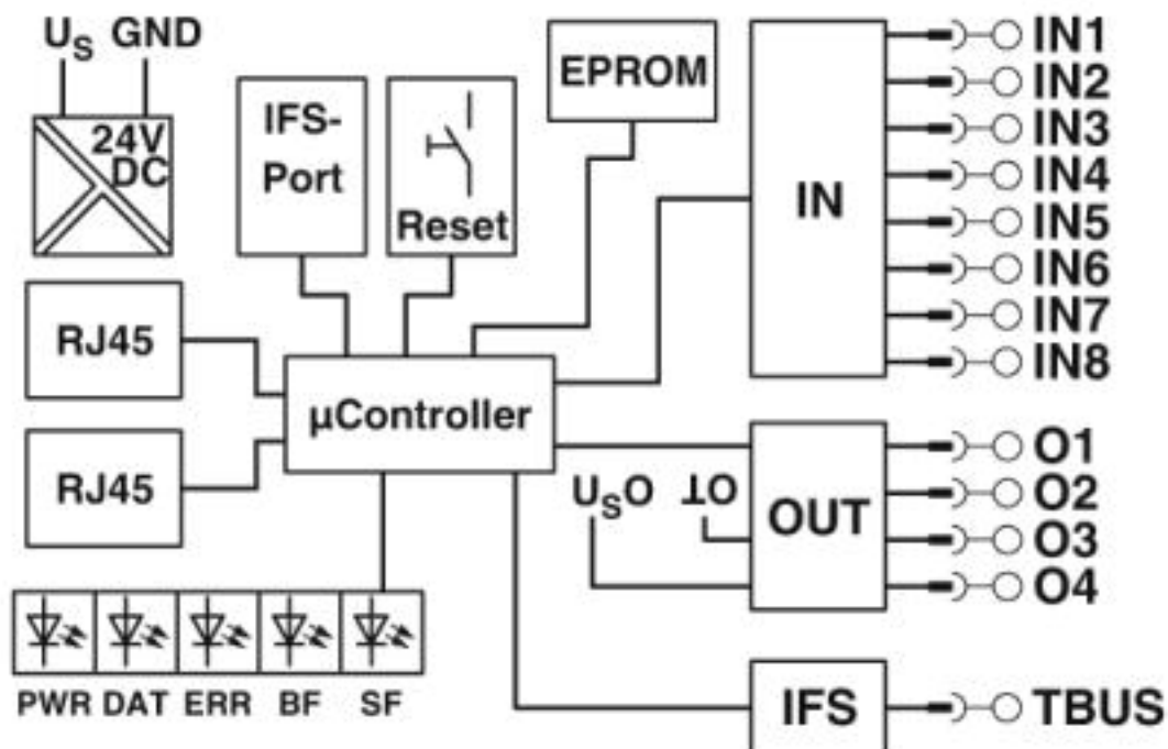
Blockschaltbild
