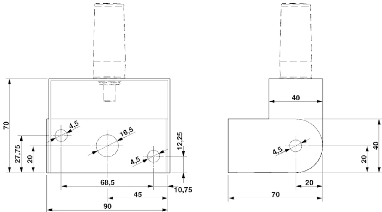
Maßzeichnung
