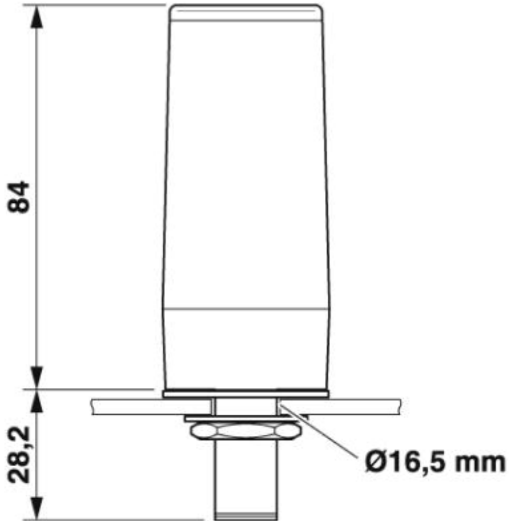
Schemazeichnung
