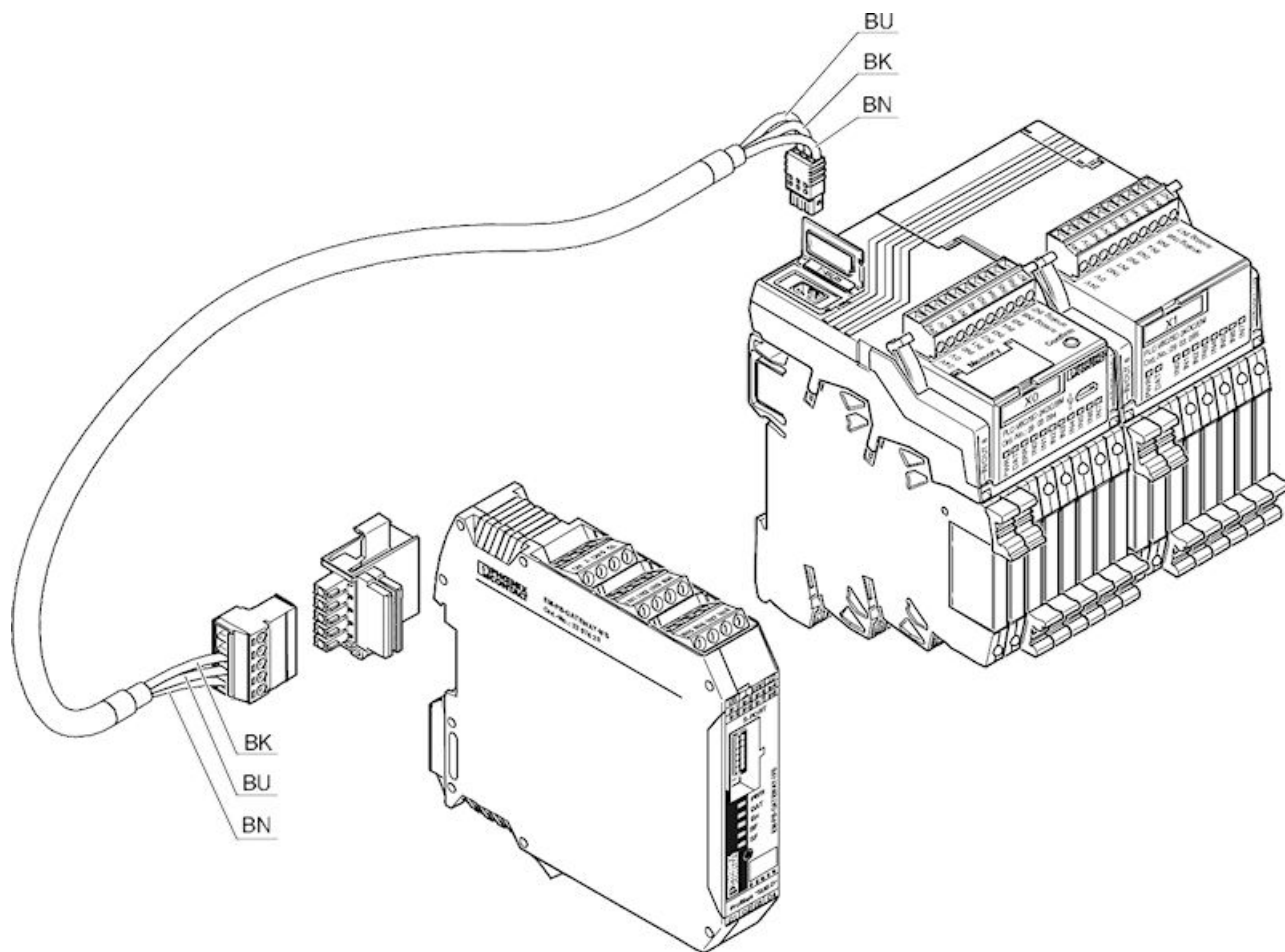
Schemazeichnung
