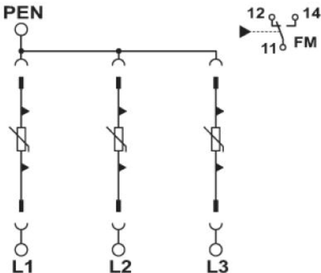
Schaltplan
