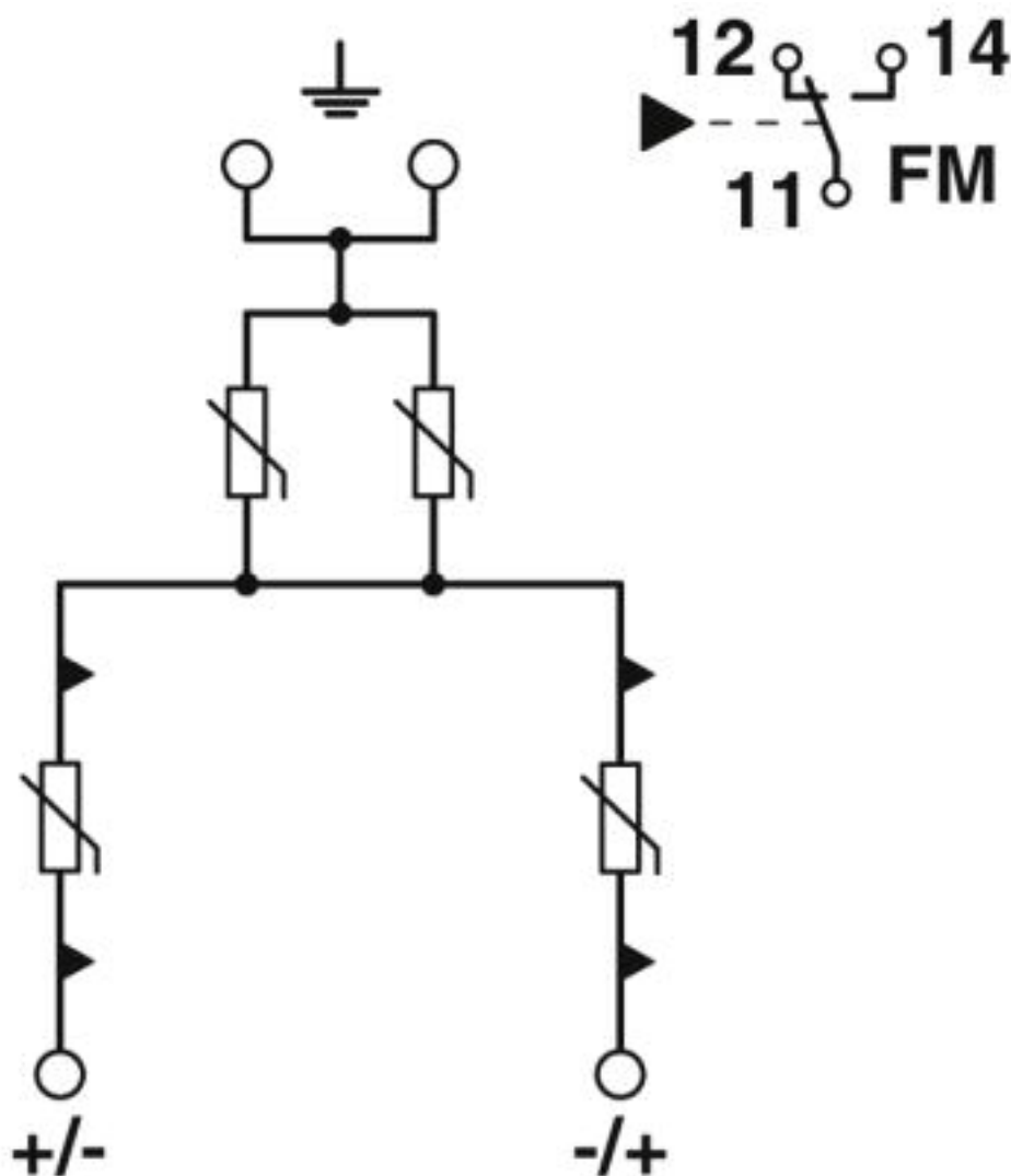
Schaltplan
