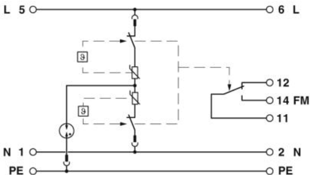
Schaltplan
