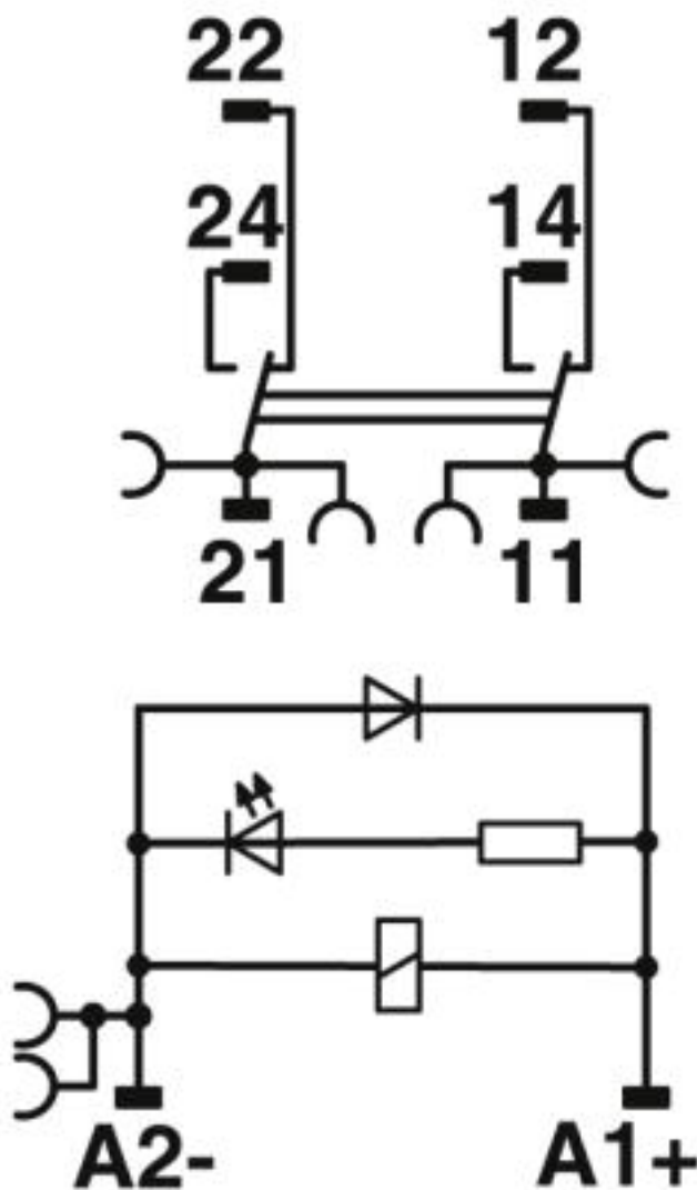
Schaltplan
