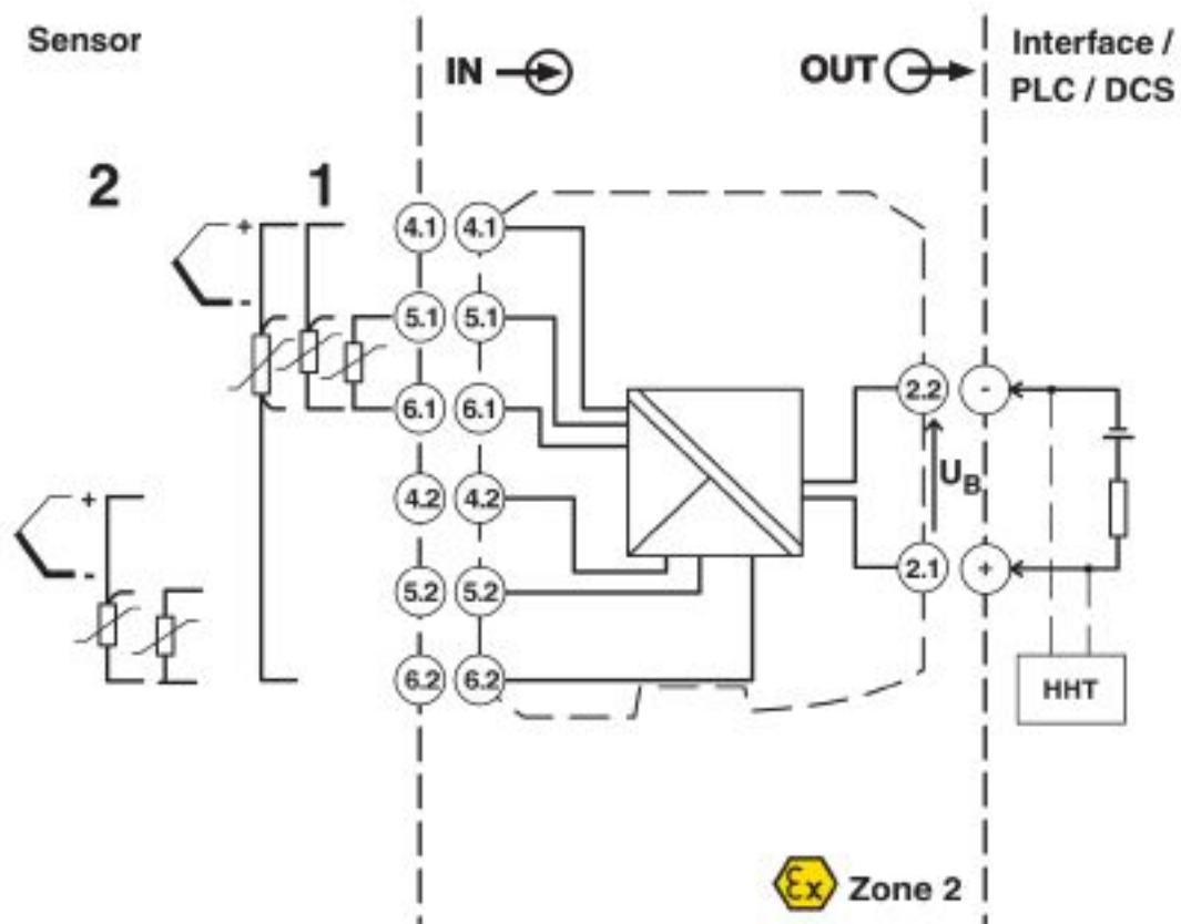
Blockschaltbild
