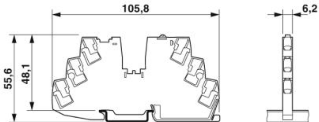
Maßzeichnung
