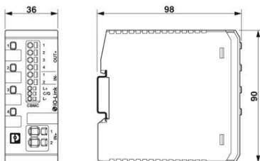
Výkres výrobku
