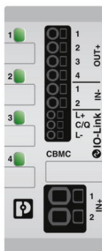
Výkres výrobku
