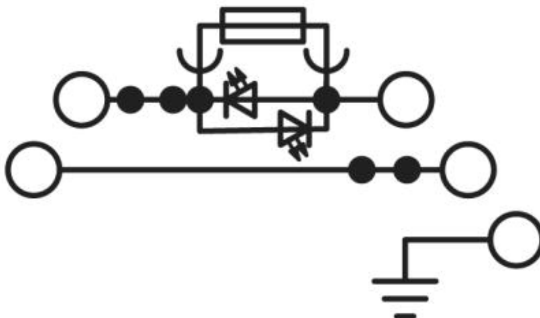
Schaltplan
