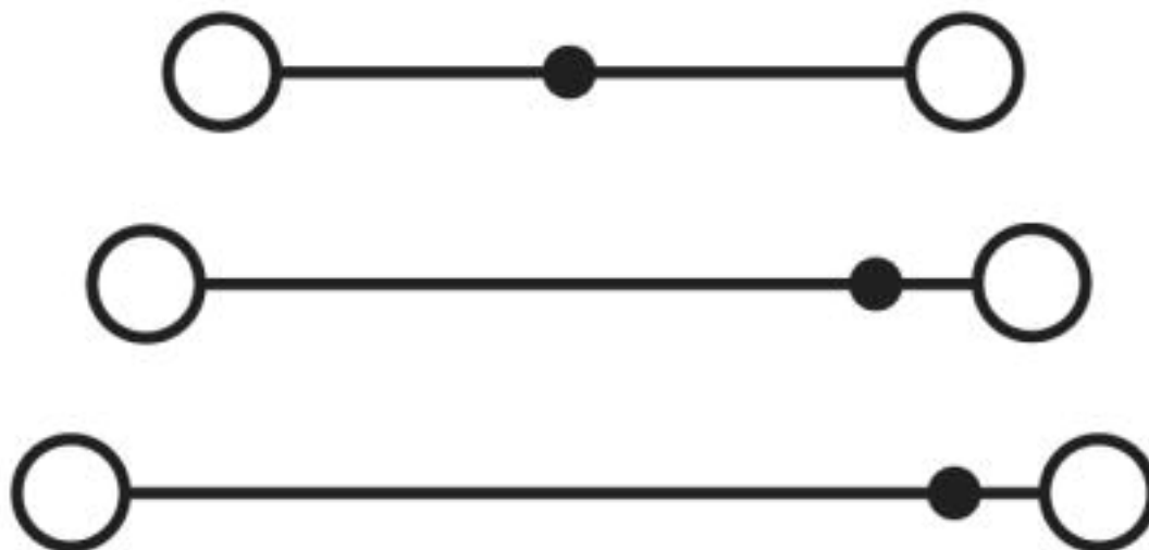
Schaltplan
