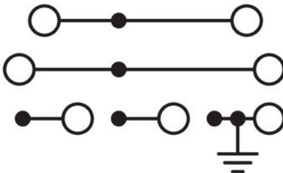
Schaltplan
