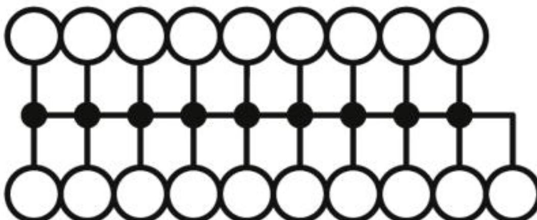
Schaltplan
