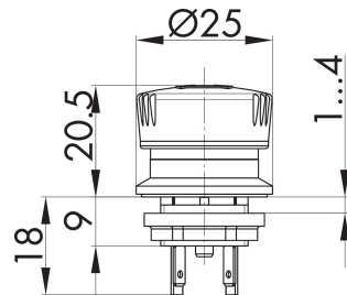
Maßskizze:
