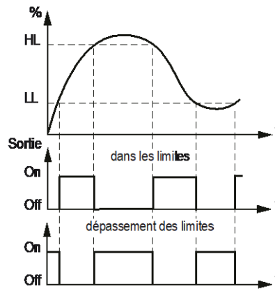
Fig. 6.2 Contrôle de sortie
