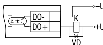
Fig. 5.6 NPN transistor Sortie
