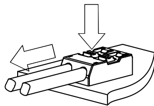
Fig. 5.3 Deconnexion du fil
