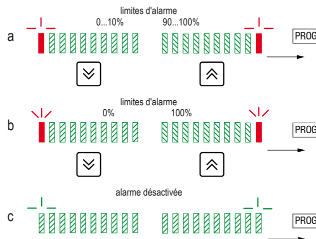
Fig. 6.4 Réglage de l'alarme aux valeurs limites
