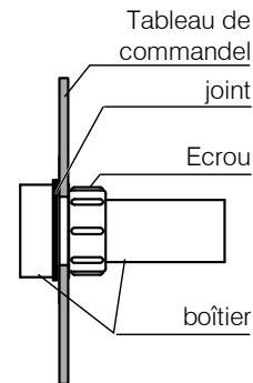
Fig. 5.4 Montage
