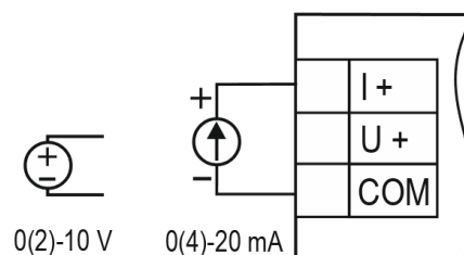
Fig. 5.5 Câblage d'entrée
