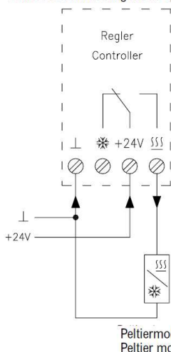
Anschluss im Heizbetrieb Connection for heating mode operation
