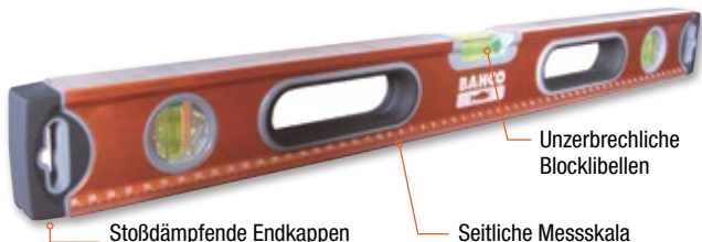
Stoßdämpfende Endkappen
