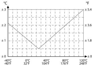
Figure 2 - Précision de la température
