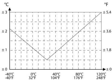
Abb. 2 – Genauigkeit der Temperatur
