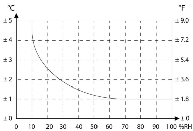
Figura 3 – Precisión del punto de rocío (a 25^{\circ}\text{C} )
