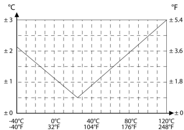
Figura 2 – Precisione della temperatura
