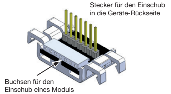
Busverbinder
