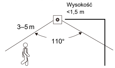
Czujnik ruchu (PIR)
