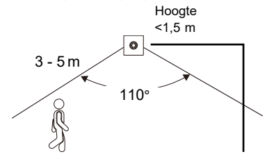
Bewegingssensor (PIR)
