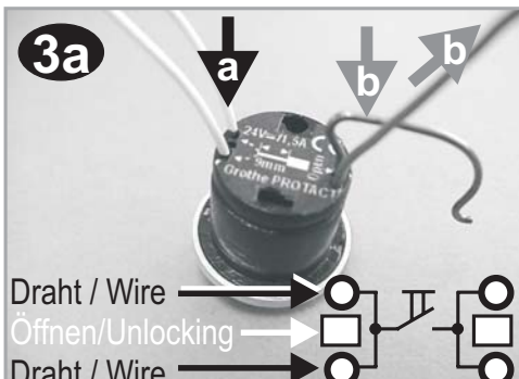
a) Verdrahtung / Wiring b) Entriegelung / Unlocking
