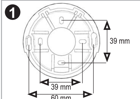
Wandbefestigung Halter Wall fixation of bracket
