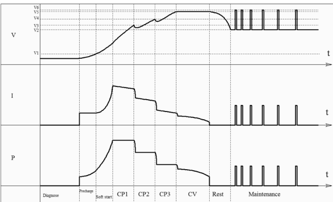
Figuur 4: Oplaadkarakteristiek voor lithiumbatterij
