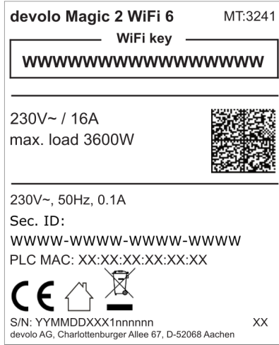
Abb. 4: landesspez. Typenschild
