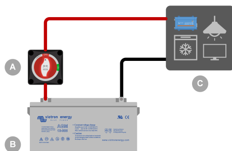
Batterieschalter zum Trennen des Haussystems von der Hausbatterie. Zur Erhaltung der Batterieladung, zur Systemwartung oder in Notfällen.
