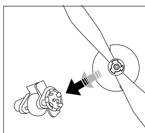
Klicken Sie den Propeller zurück in die Klammer. Setzen Sie ihn dazu schräg an.
