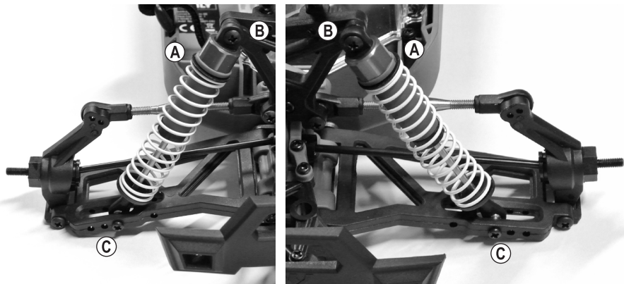
Vorderachse
