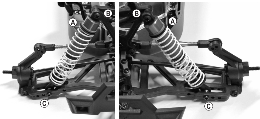
Essieu avant
