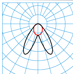
C-Line DA LED8000-830 EB3 TX046737
