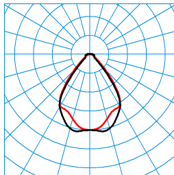
C-Line TB LED8000-840 05 TX055460
