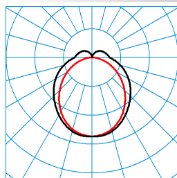
C-Line OTR LED4000-830 TX055342
