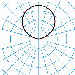
Parelia H-L 13000-840 +LM1 01 (indirect) TX059626 ■ C0 - C180 ■ C90 - C270 DIN 5040: E03 UTE: 0,00 J + 1,00 T CEN Flux Code: 0 0 0 0 100 49 82 98 100
