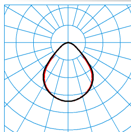
Opendo D2-L PW19 47-840 01 TX277471
