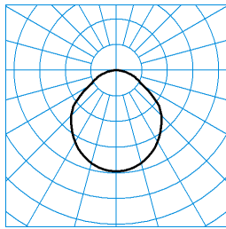
Inplana C11 OTA25 5000-840 01 TX057258
