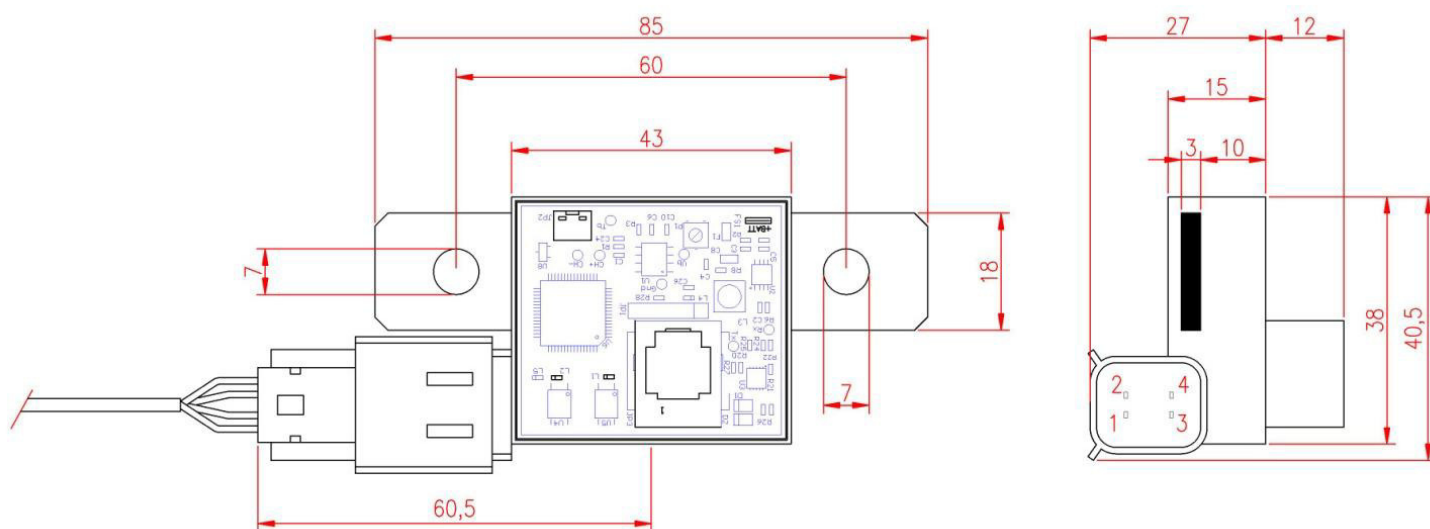
Fig.6 - Dimensioni WBM
