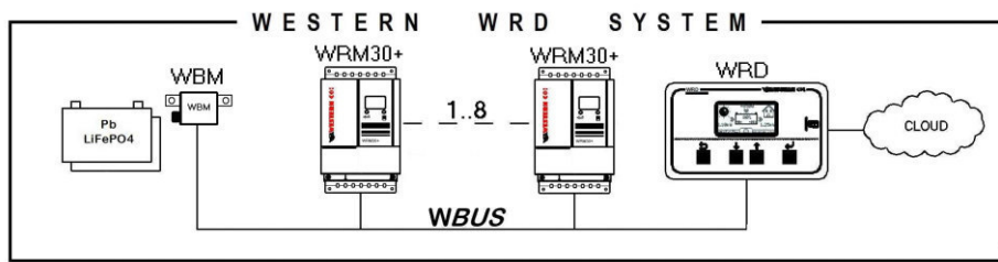
Abb. 1 WESTERN WRD SYSTEM mit WRM30+
