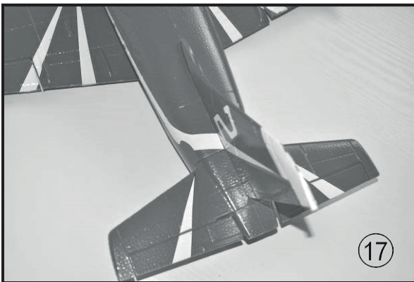
Bild 17 – Kleben Sie das Seitenleitwerk in den Rumpf. Achten Sie darauf, dass es gerade zum Rumpf ausgerichtet ist.
