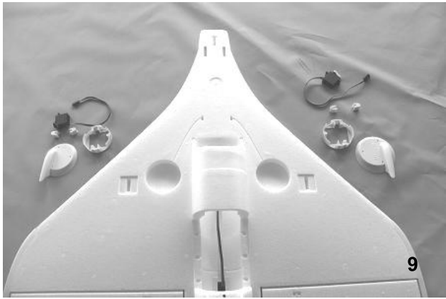
Bild 9 – Benötigt werden Querruder Servos, Halterung und Abdeckung.
