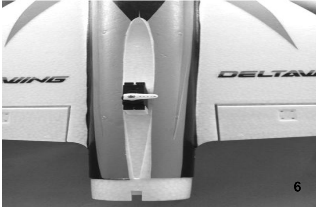
Bild 6 – Montieren Sie den Servo.
