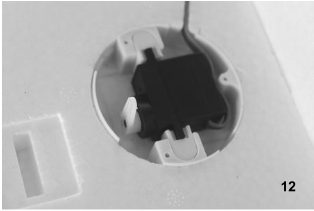
Fig. 12 - Install the servo.
