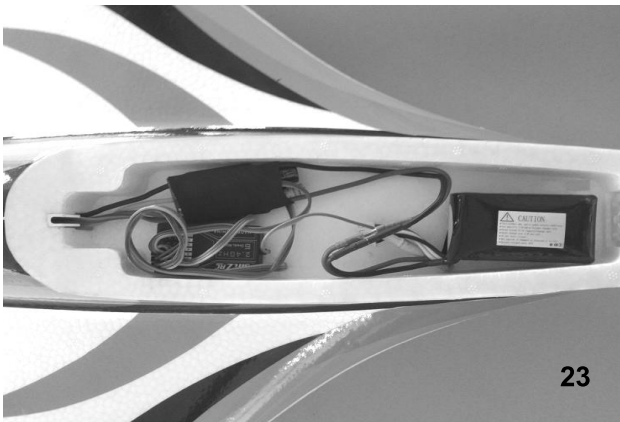
Bild 23 – Schließen Sie den ESC und die Servos am Empfänger an. Beachten Sie dazu die Angaben zur Kanalbelegung in der Anleitung des Sender-Herstellers. Positionieren Sie den Akku. Laden Sie den Akku bevor Sie ihn anschließen.
