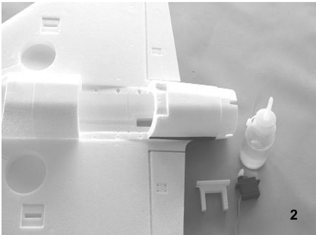
Bild 2 – Benötigt werden Servo und Servohalterung.
