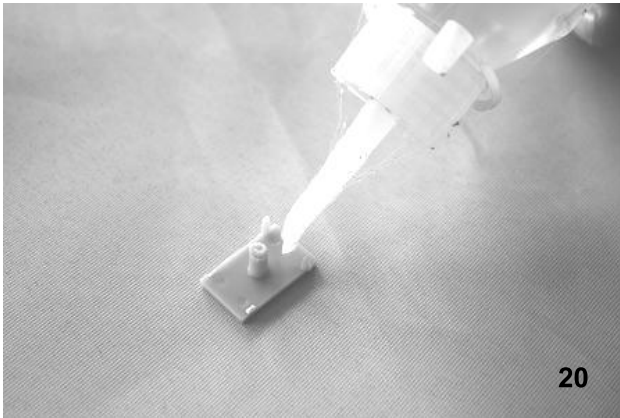
Bild 20 – Bringen Sie Kleber am Verschlusssteil an.
