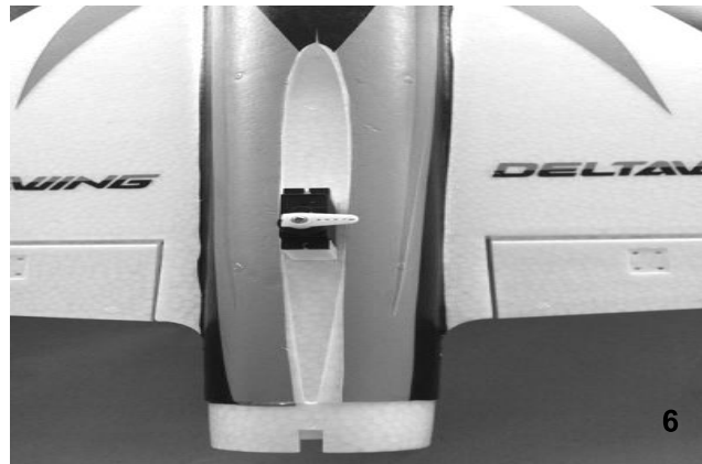
Fig. 6 - Install the rudder servo.
