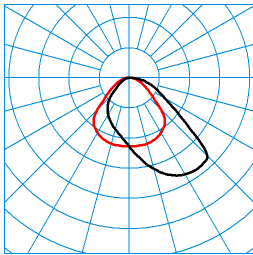
Cultega Act T COM PAW 600 ETDI KL 05 (ACTDCW) TX280841 ■ C0 - C180 ■ C90 - C270 DIN 5040: A40 UTE: 1,00 D CEN Flux Code: 54 85 97 100 100
